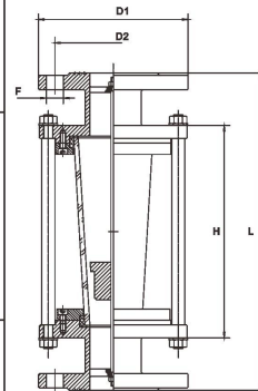
Fa100外形尺寸图
