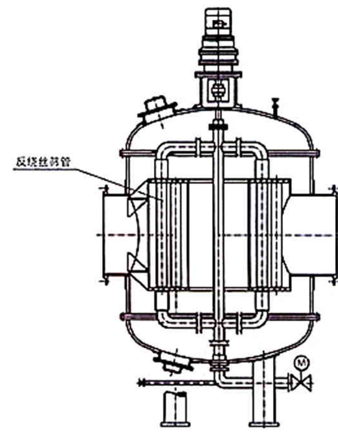
反绕筛管工作图
